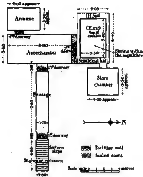
مسقط أفقى لقبرة توت عنخ آمون كما رسمه هوارد كارتر
